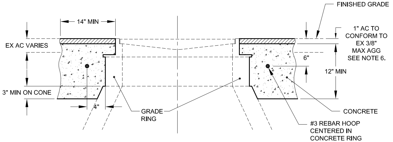
MANHOLE & RISER
